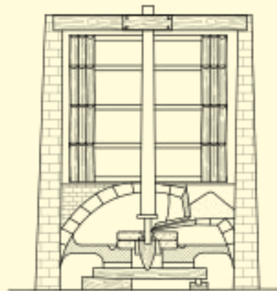
Eolienne à axe vertical
